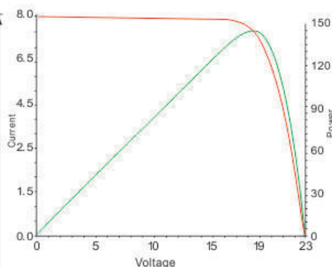
IV测试曲线
