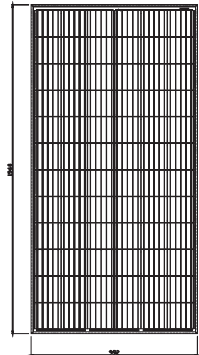
Module Front Side
