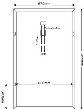
Module Diagram
