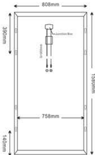
Module Diagram
