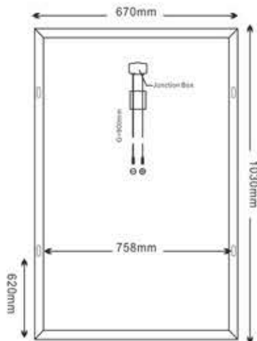
Module Diagram
