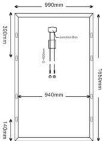
Module Diagram
