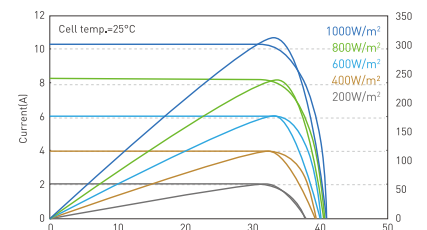
不同辐照度下电流电压曲线 / 功率电压曲线 (315W)
