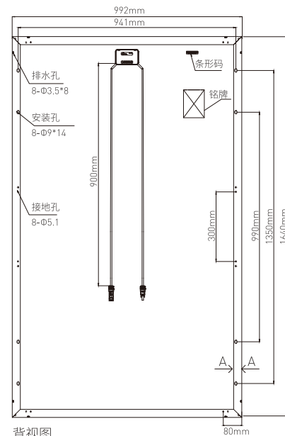
背视图
