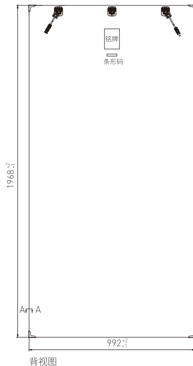
背视图
