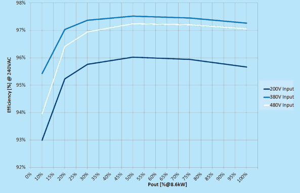
UNO-8.6-TL-OUTD-S-US
