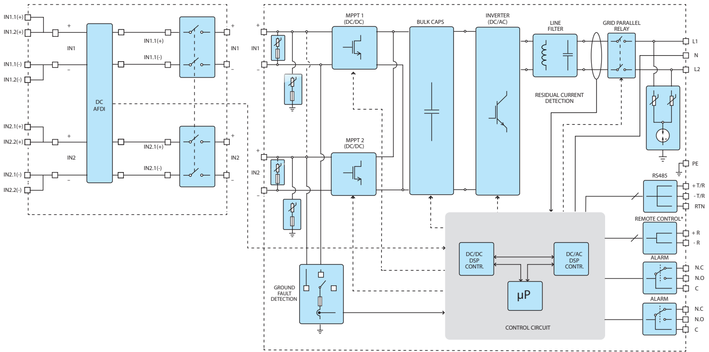
UNO-7.6-TL-OUTD-S-US
