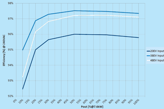
UNO-7.6-TL-OUTD-S-US
