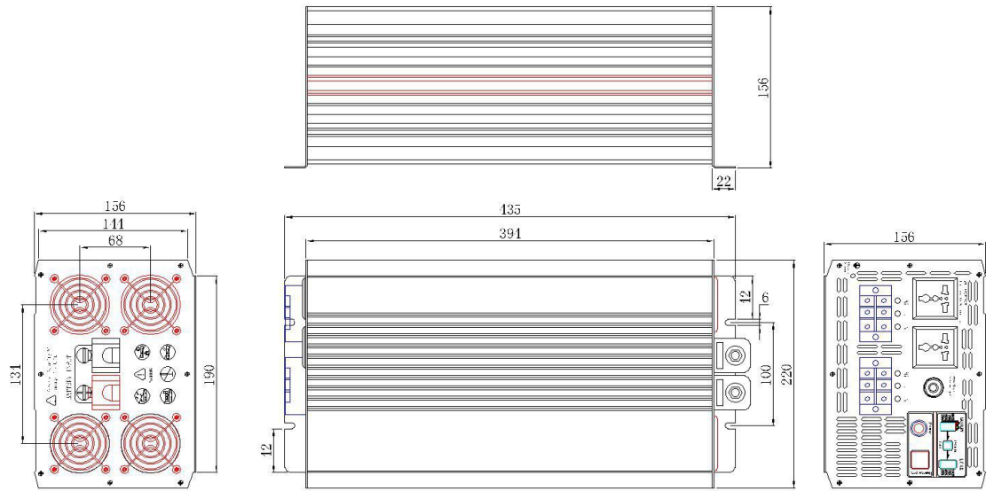
4000W纯正弦波外壳结构图
