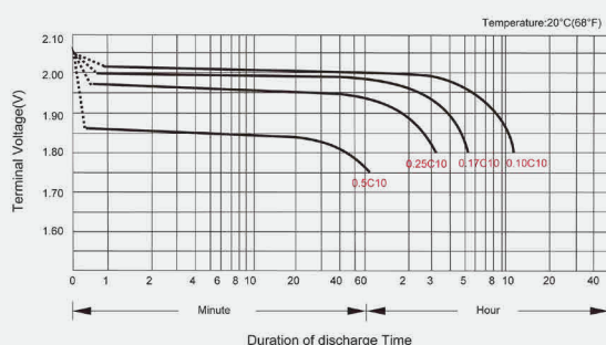
放电曲线 Discharge Characteristics
