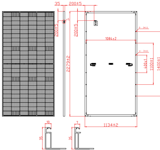
边框截面图
