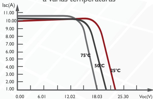
Curva I-V de módulo SAYA-M210-36 a varias temperaturas
