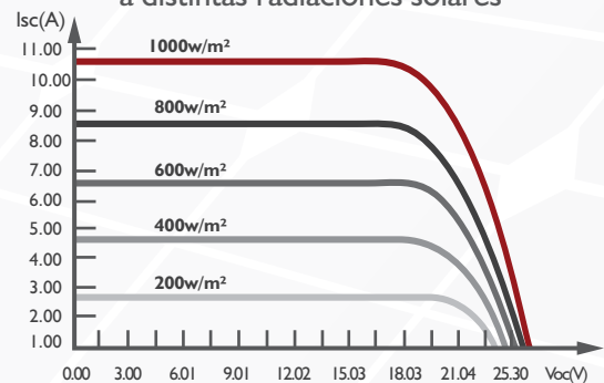
Curva I-V de módulo SAYA-M210-36 a distintas radiaciones solares
