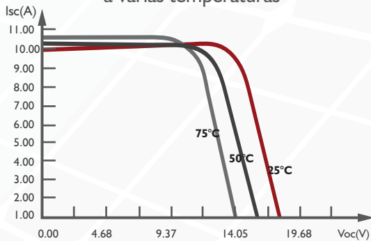
Curva I-V de módulo SAYA-M165-28 a varias temperaturas
