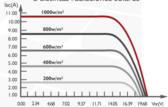
Curva I-V de módulo SAYA-M165-28 a distintas radiaciones solares
