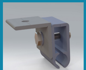
4. Calzip Clamp
