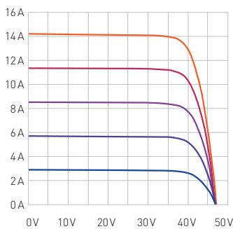
■ 1000 W/m 2 ■ 600 W/m 2 ■ 200 W/m 2 ■ 800 W/m 2 ■ 400 W/m 2
