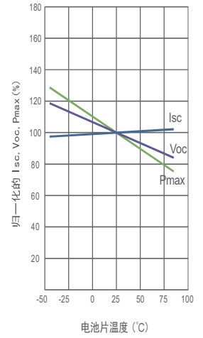
Isc, Voc, Pmax的温度曲线
