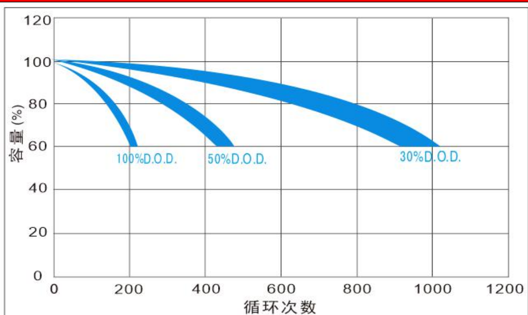
使用寿命与放电深度的关系(25°C/77°F)
