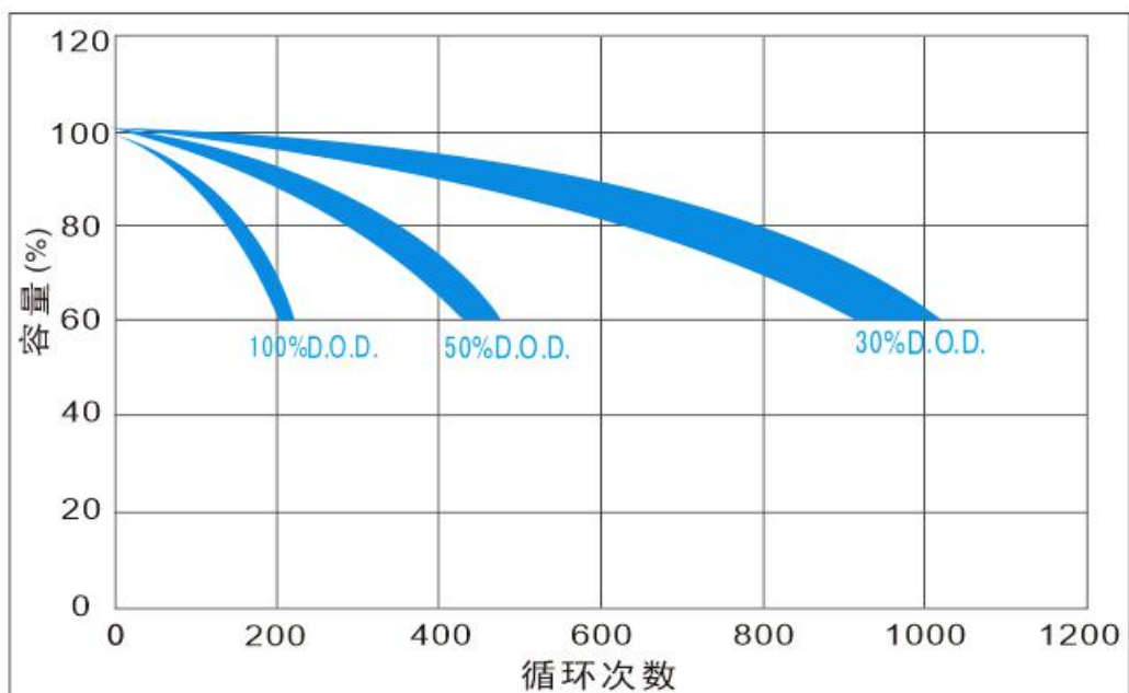
使用寿命与放电深度的关系(25°C/77°F)
