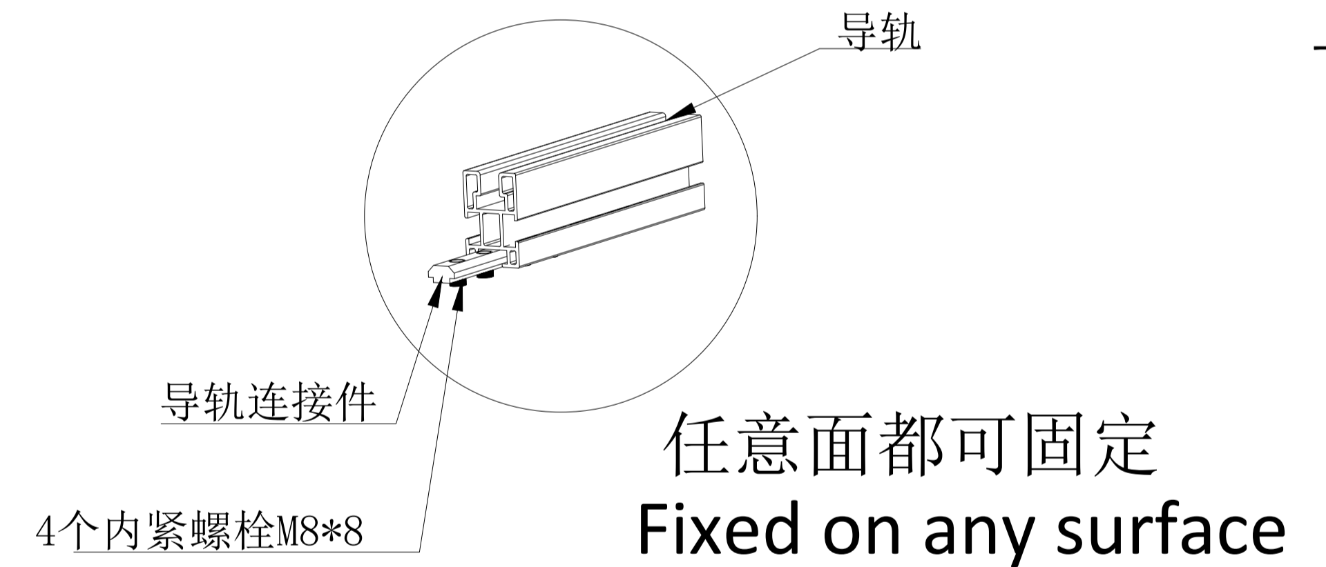
导轨连接件安装示意图 Installation of guide rail connectors
