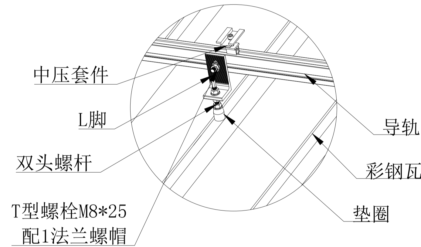
L脚安装示意图 L-feet installation
