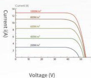
I-V CURVE(455W)
