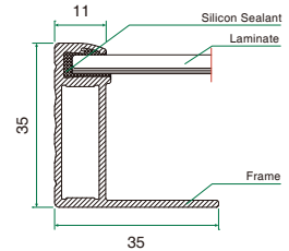
(A-A)
