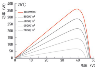
功率-电压曲线 (JD360M6P-36)
