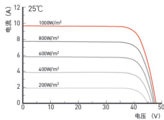
电流-电压曲线 (JD360M6P-36)
