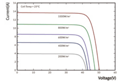
I-V曲线
