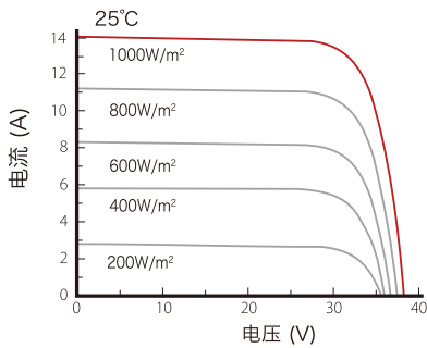
电流-电压曲线 OLV-410-54M-HEAH
