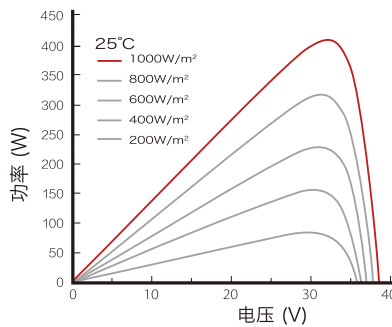
功率-电压曲线 OLV-410-54M-HEAH
