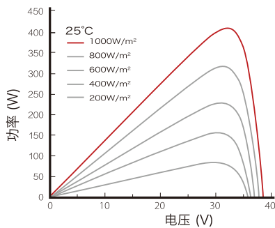
功率-电压曲线 OLV-410-54M-DEAH
