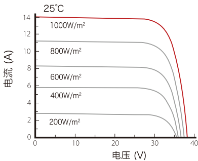
电流-电压曲线 OLV-410-54M-DEAH
