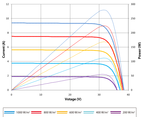
电流-电压 & 功率-电压曲线图 (280)
