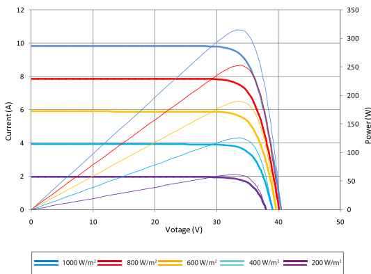
电流-电压 & 功率-电压曲线图 (320W)
