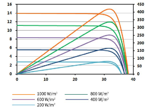
功率-电压&电流-电压曲线
