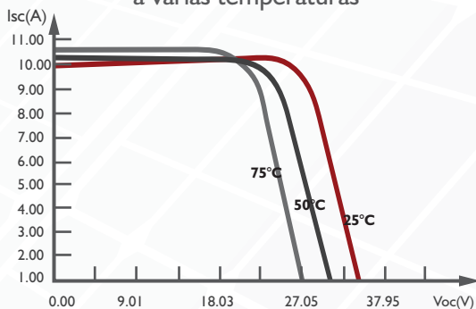
Curva I-V de módulo SAYA-M315-54 a varias temperaturas
