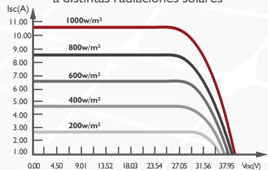
Curva I-V de módulo SAYA-M315-54 a distintas radiaciones solares
