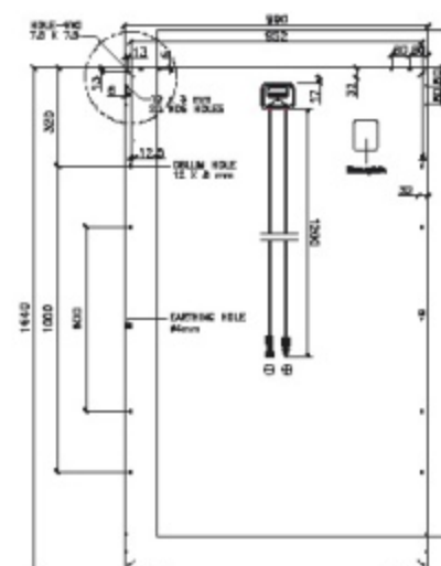
DIMENSIONS/ DIMENSIONES ESF-270PA
