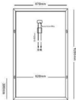
Module Diagram
