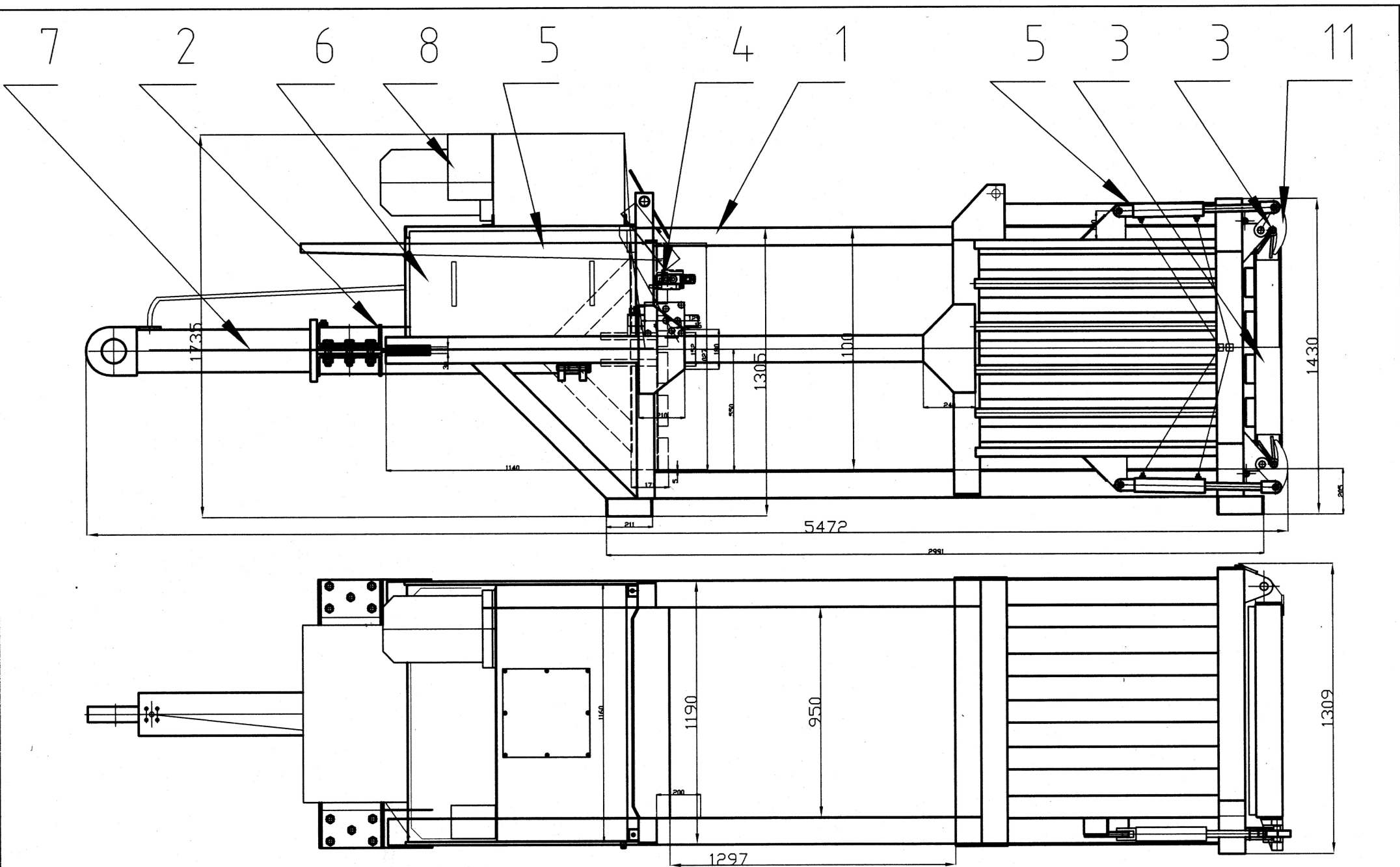
Габаритный чертеж прессы ПГ-50
